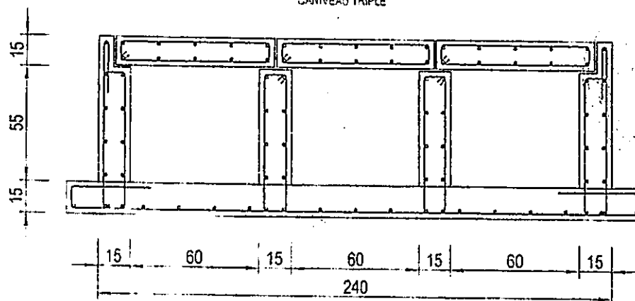
CANIVEAU TRIPLE
